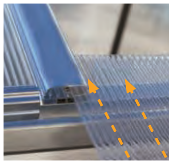
A táblák egyszerűen rögzíthetők a kerületi profilokban.
